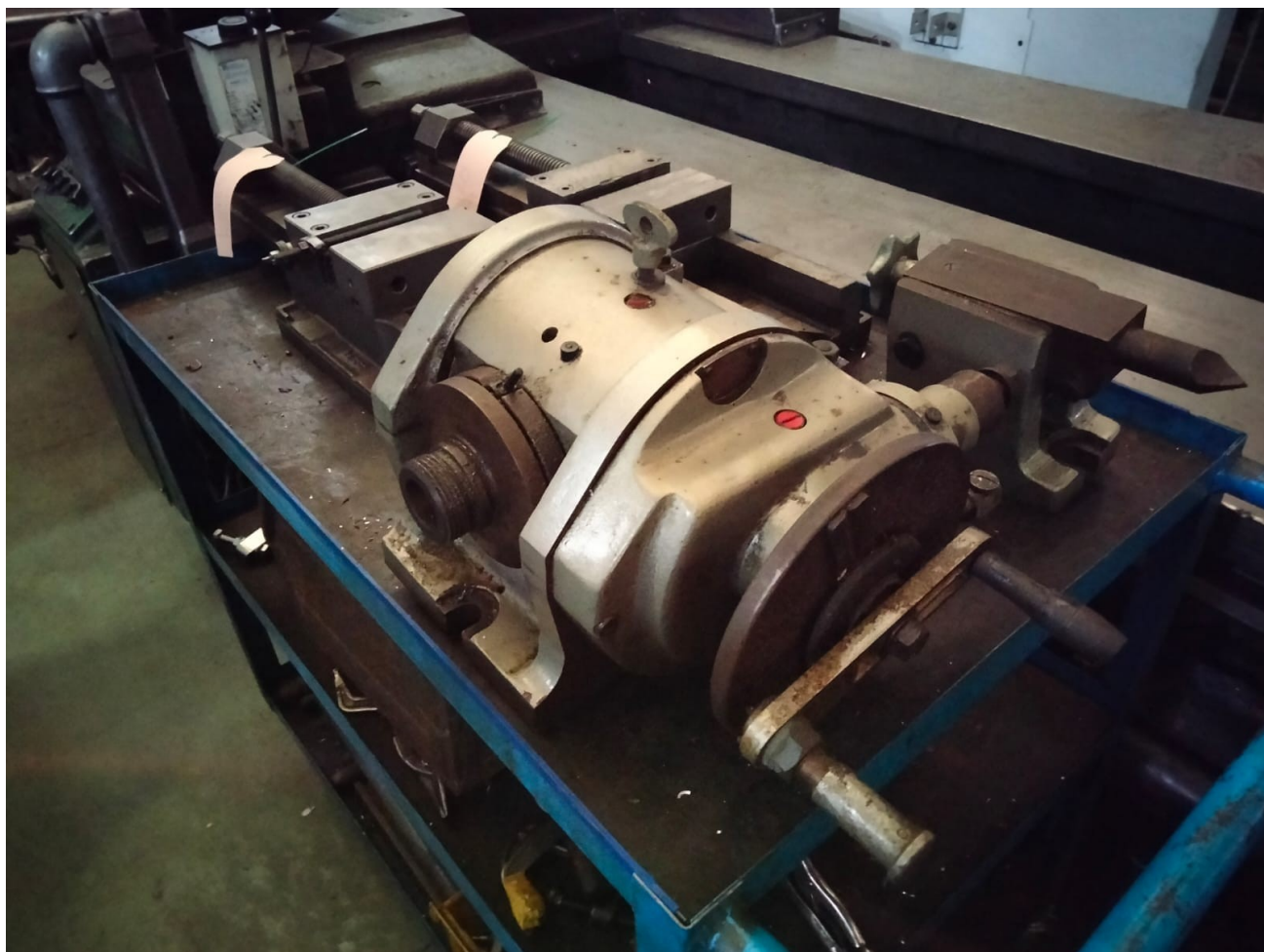
10973 DIVISORE CON CONTROPUNTA
